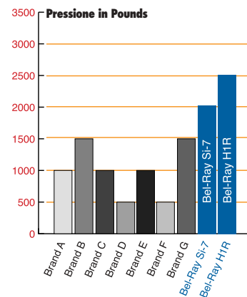
Figura A: Bel-Ray H1R e Si-7 confronto con altre gamme di olio per motori da corsa a 2 tempi.
